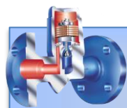
CONA®-B Биметаллические конденсатоотводчики
