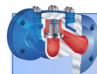
CHECKO®-V Обратные клапаны подъемные
