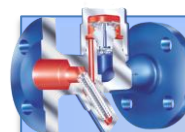
CONA®-M Мембранные конденсатоотводчики
