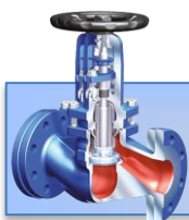
FABA®-Plus / -Supra Запорные клапаны с сильфонным уплотнением
